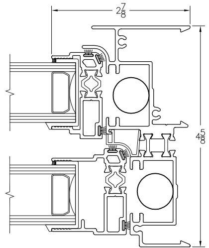
4 JAMB
