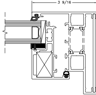
OPERABLE JAMB
