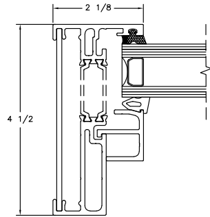
FIXED JAMB
